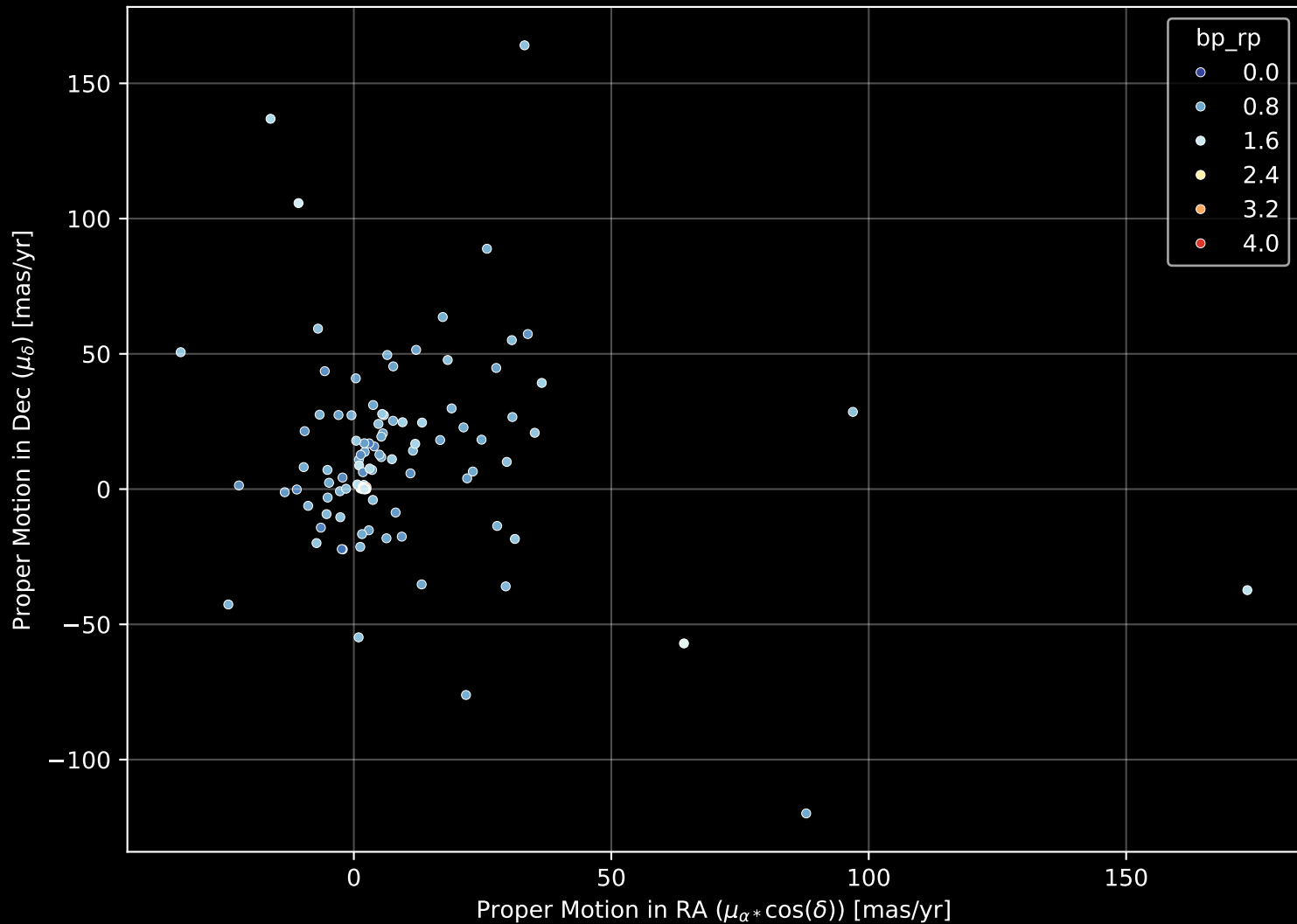
APOGEE DR17 Field: [281-34-O] Proper Motion Diagram (n= 147)
