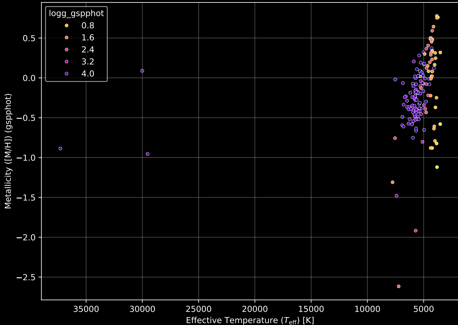
APOGEE DR17 Field: [281-34-O] Stellar Population Parameters (n= 147)
