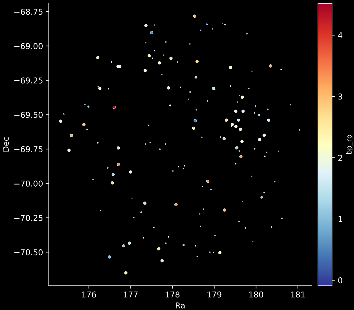
APOGEE DR17 Field: [281-34-O] Stars: 147
